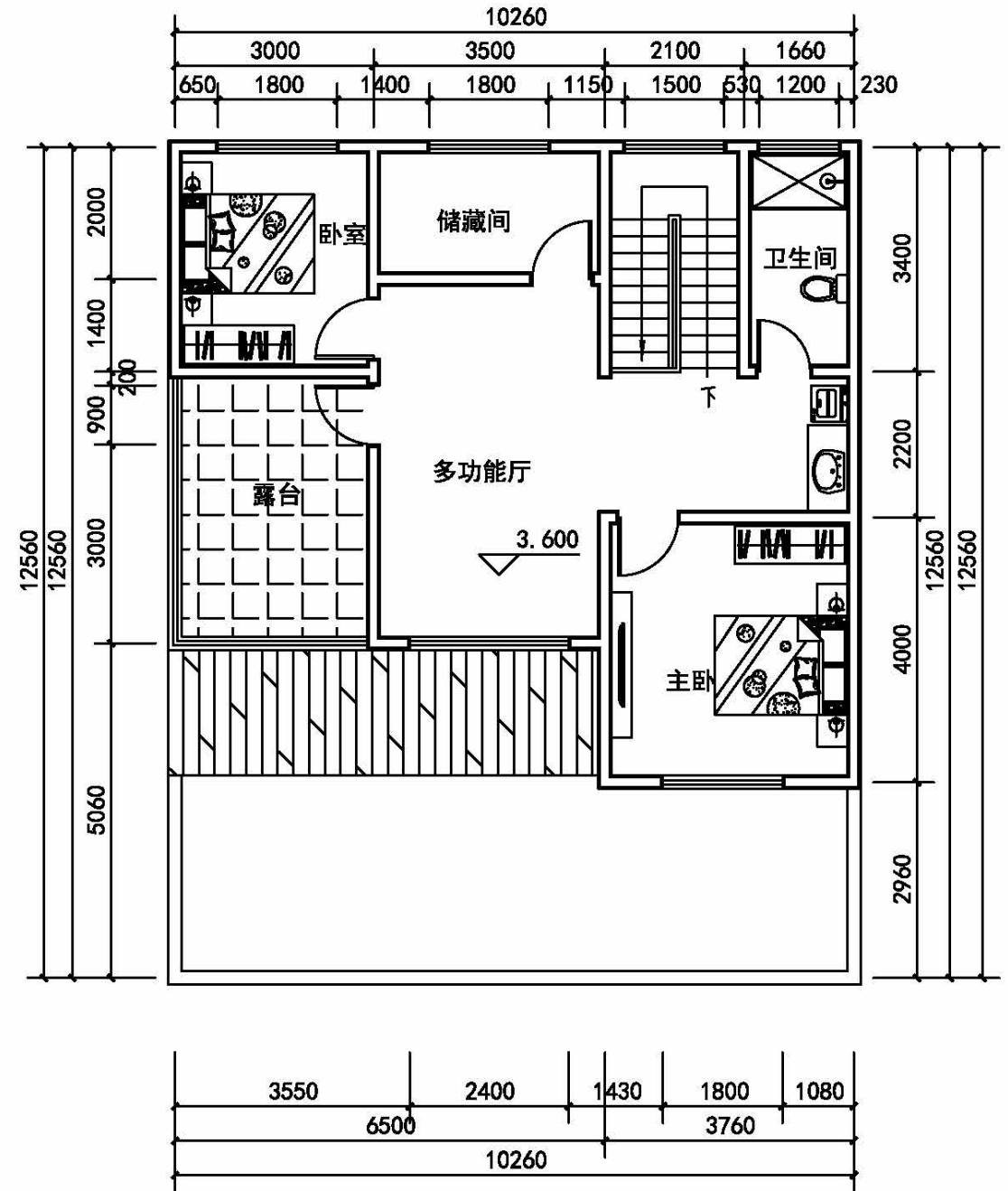
二层平面图 1:100
