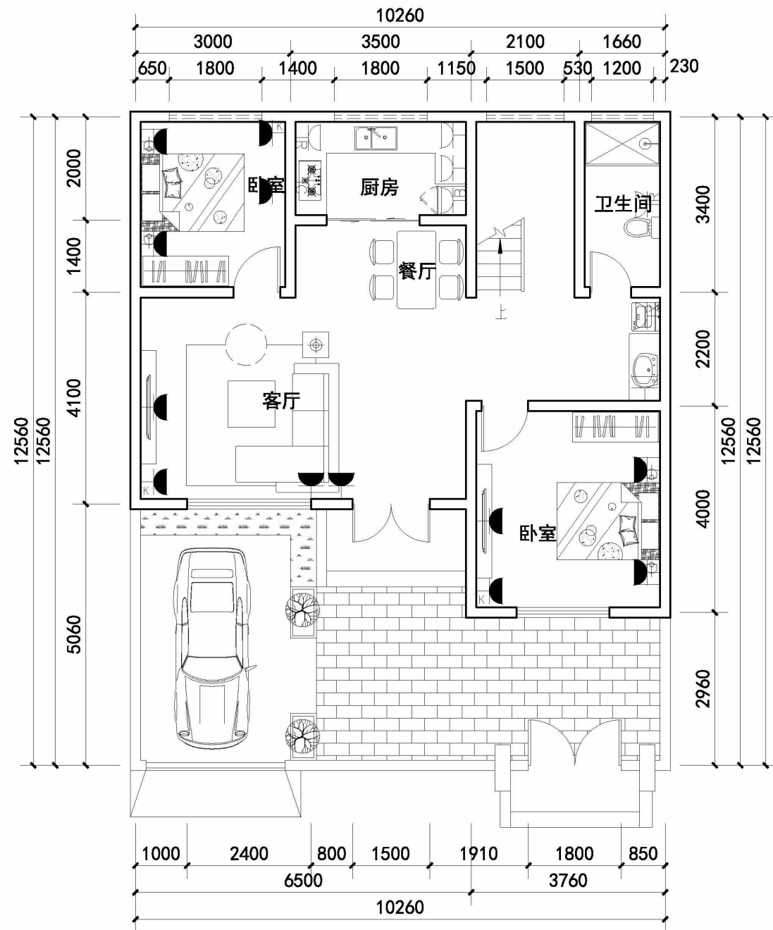
一层插座平面图 1:100
