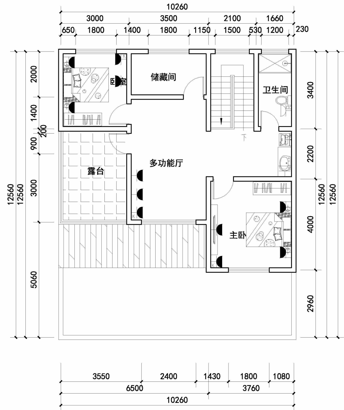
二层插座平面图 1:100
