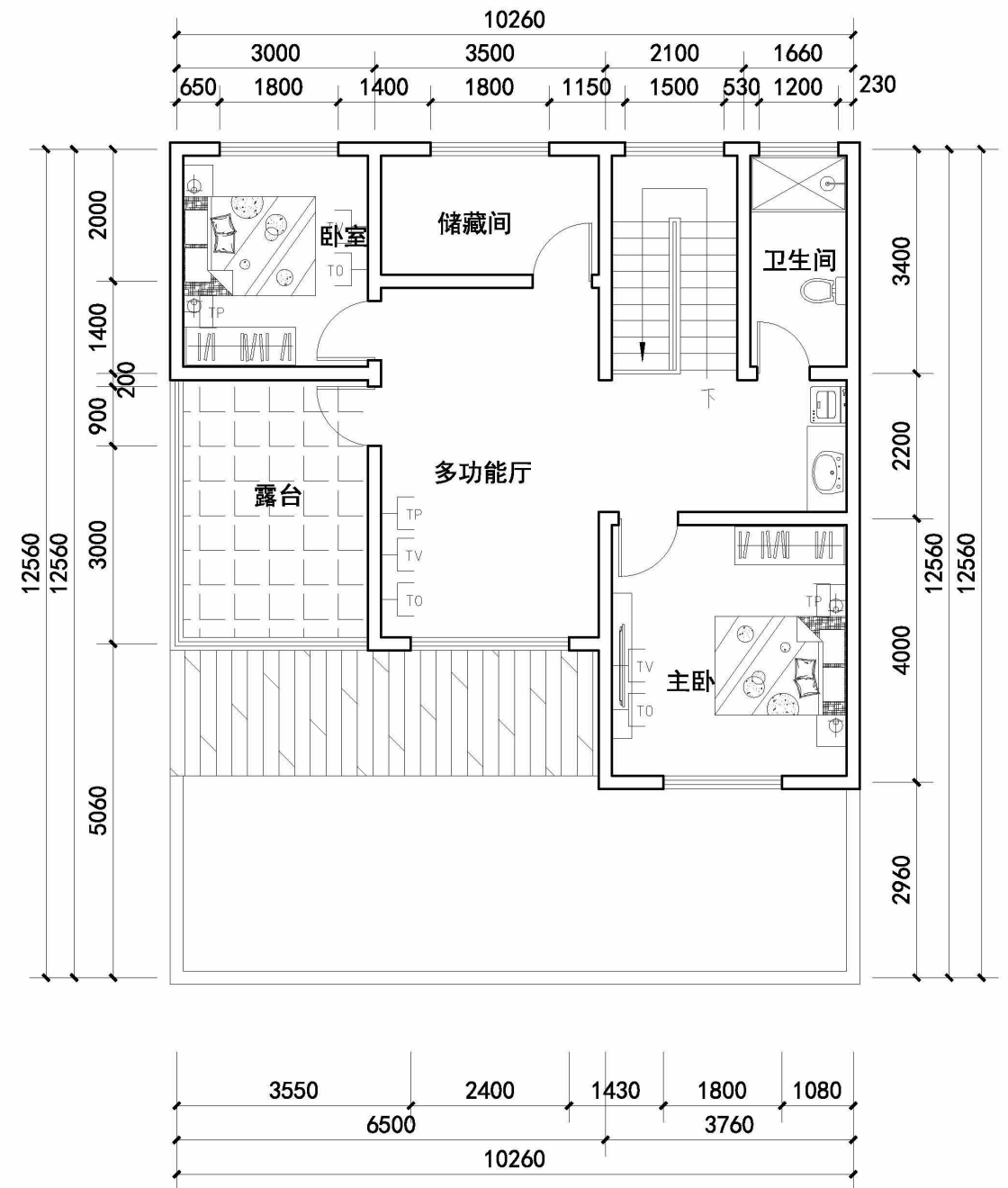
二层弱电平面图 1:100
